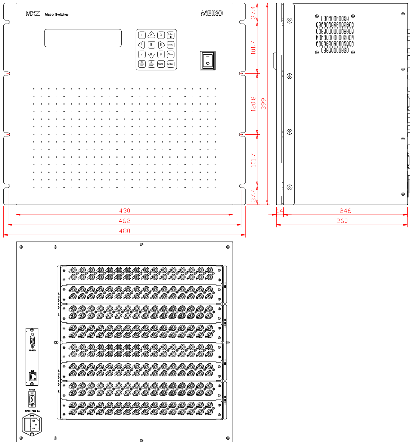
MXZ64-64A (ラックマウント金具実装図)
