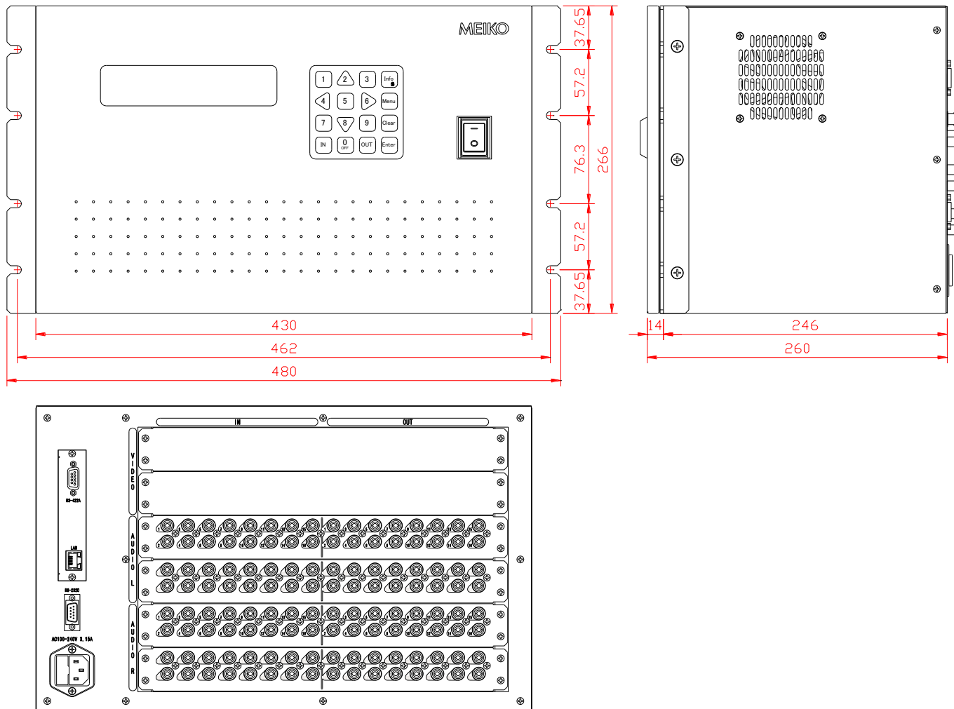
MXZ32-32A (ラックマウント金具実装図)
