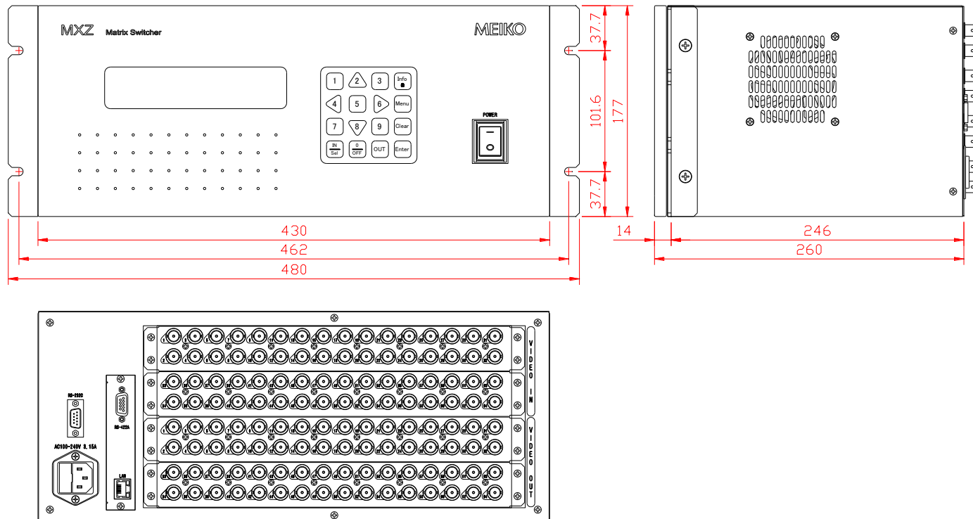
MXZ64-64V（ラックマウント金具実装図）
