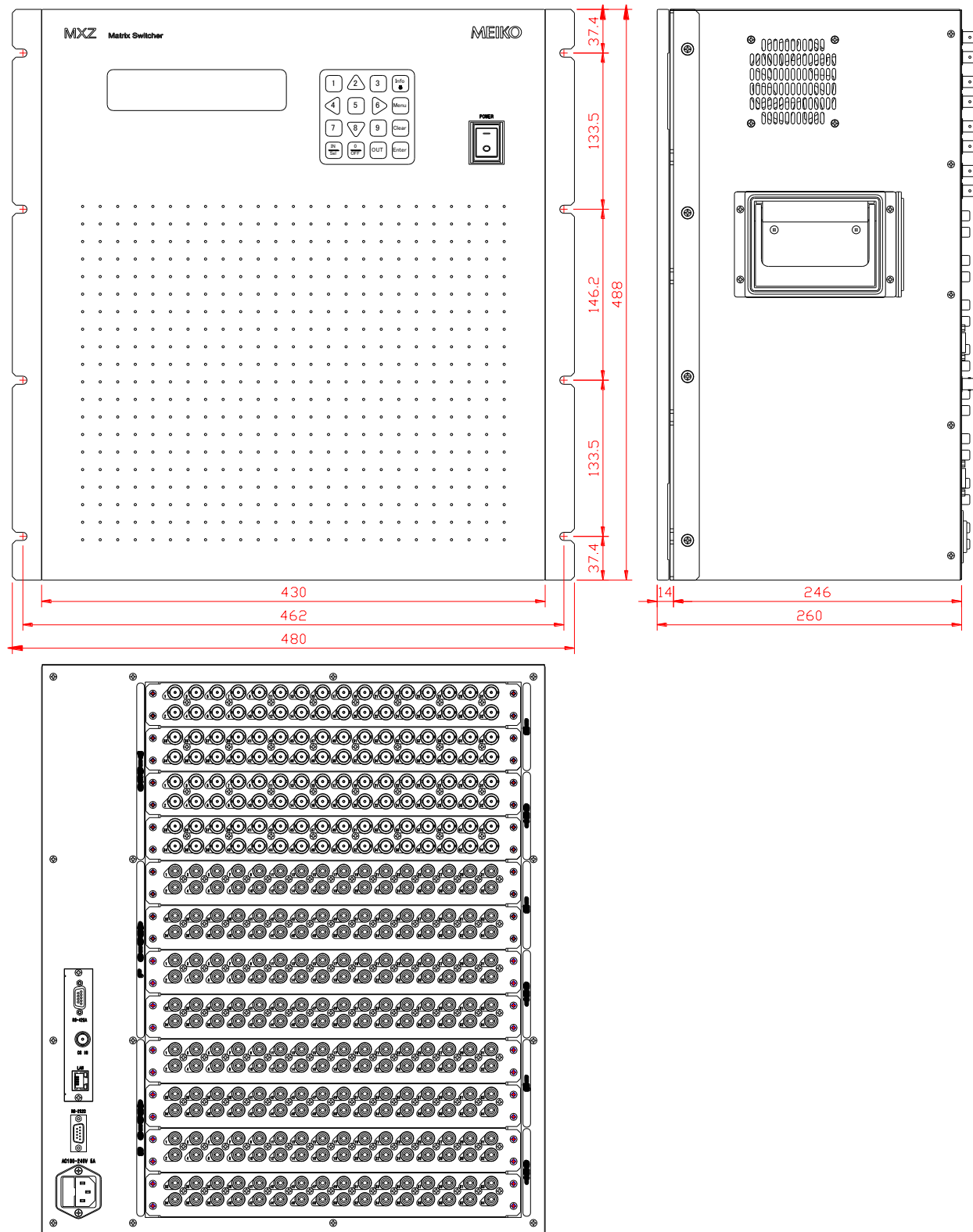
MXZ64-64AV (ラックマウント金具実装図)
