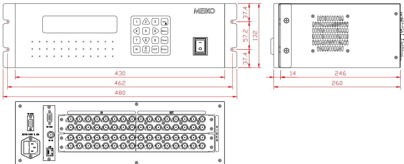
MXZ32-32V（ラックマウント金具実装図）
